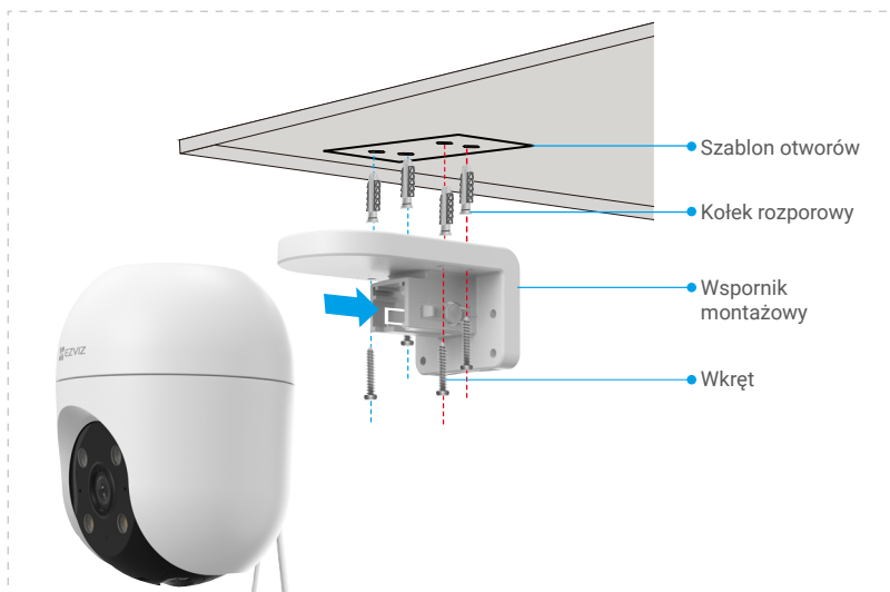
Rys. 1 Montaż sufitowy
