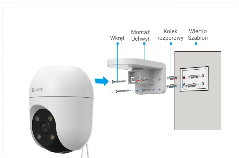
Rys. 2 Montaż ścienny
